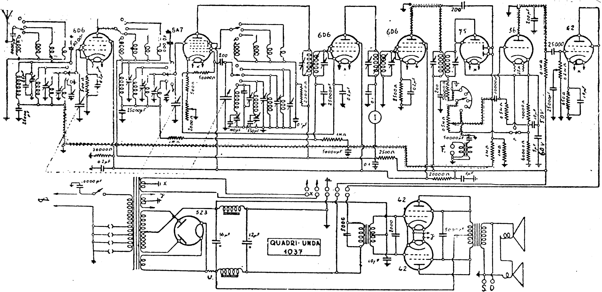
UNDA RADIO — Mod « Quadri Unda 1037 Radiofono ». - Produzione 1937 Media frequenza. 450 kHz
